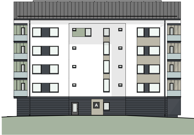
JULKISIVU KOILLISEEN / Keskuskujalle
