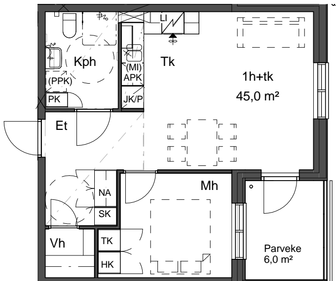
Asuntotyyppi 3 1 : 100
