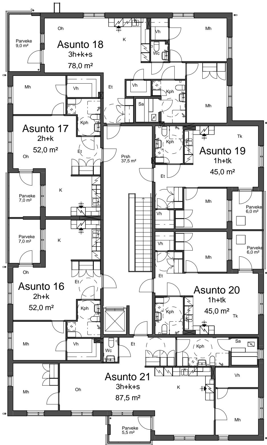
4. krs 1 : 150
