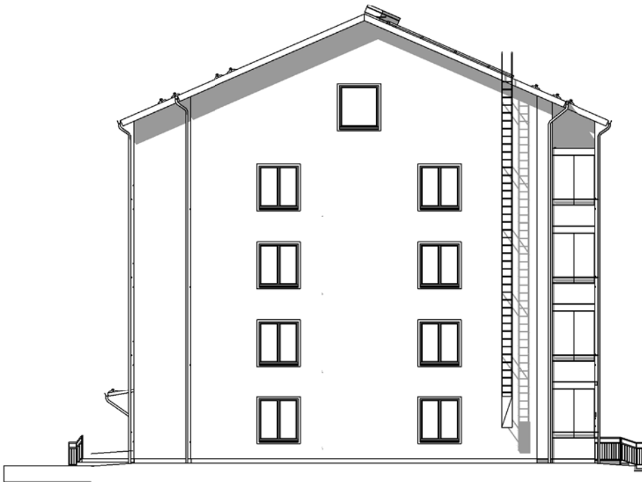
Julkisivu pohjoiseen
